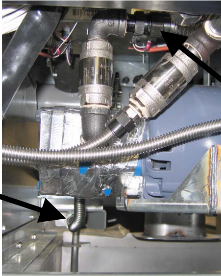
Déconnexion des conduits flexibles indiqués par les flèches.
