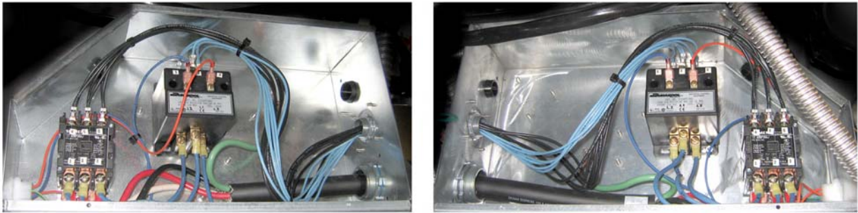
Vues gauche et droite des composants des boîtiers de contacteurs mécaniques
